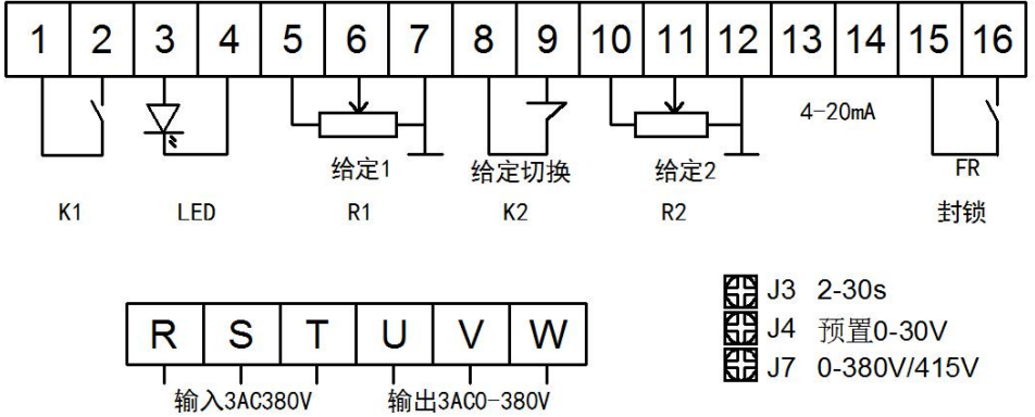
KTS 系列新型数字力矩电机控制器接线图
